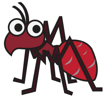
ANT
